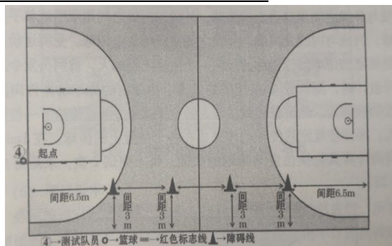
(图 1 全场综合运球上篮测试场地示意图)
